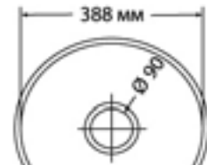
вид сверху
