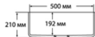
боковое сечение
