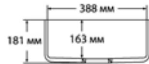
боковое сечение
