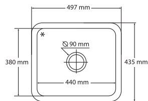
вид сверху
