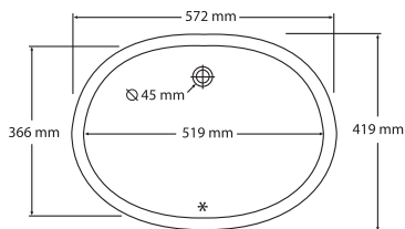
вид сверху
